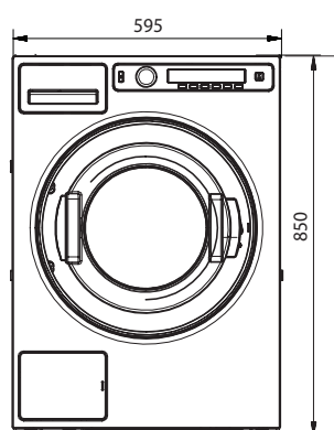
SC70 Devant
